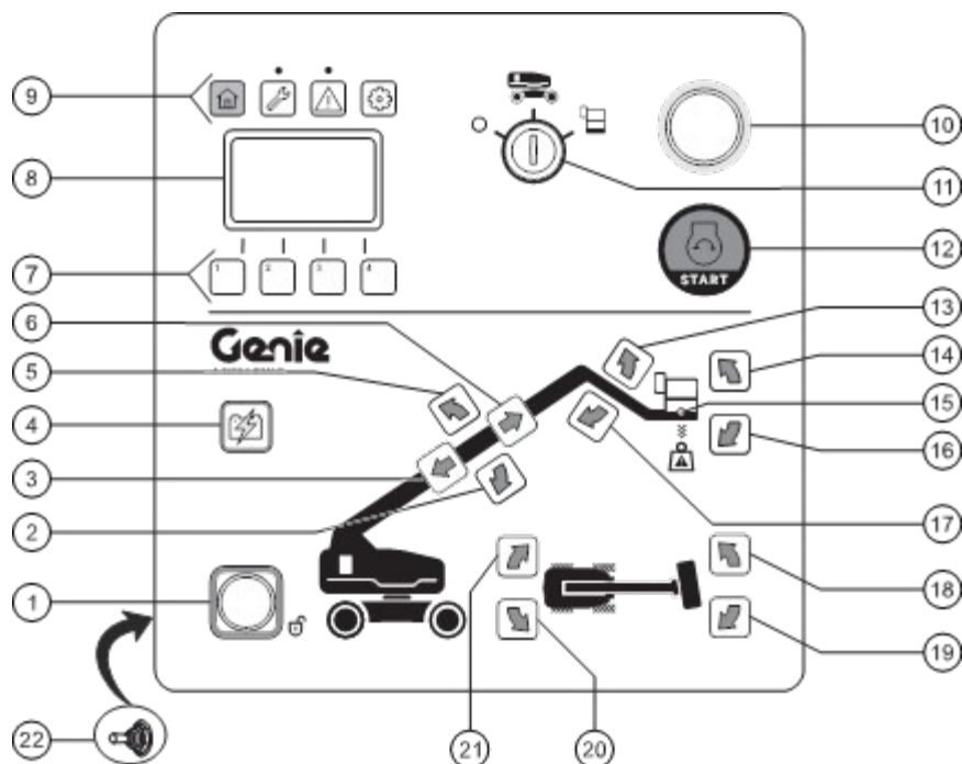
Panoul de comandă de la nivelul solului
